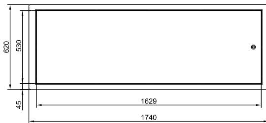
Boven aanzicht
