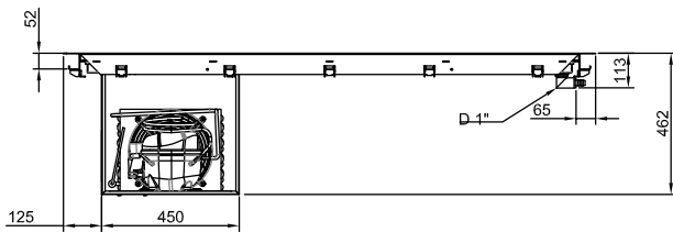
Zij aanzicht
